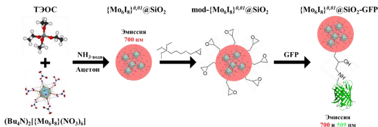
Рис. 22. Схема получения конъюгата \{\text{Mo}_6\text{I}_8\}^{0,01} @ \text{SiO}_2\text{-GFP}
