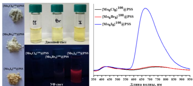
Рис. 13. Спектры люминесценции порошковых образцов \{\text{Mo}_6\text{X}_8\}^{100}@\text{PSS}
