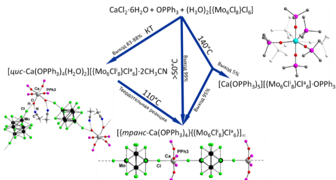
Рис. 11. Схематичное представление химических превращений в системе \text{Ca}^{2+} , [\{\text{Mo}_6\text{Cl}_8\}\text{Cl}_6]^{2-} и трифенилфосфиноксид
