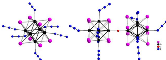
Рис. 10. Структура кластерного комплекса [\{\text{Mo}_6\text{I}_8\}(\text{N}_3)_6]^{2-} (слева) и [\{\{\text{Mo}_6\text{I}_8\}(\text{N}_3)_5\}_2\text{O}^{a-a}]^{4-} (справа)
