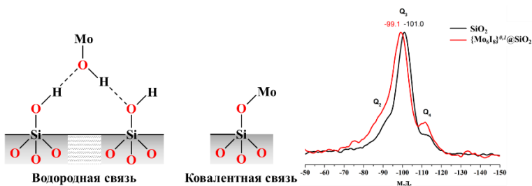
Рис. 19. Возможные типы взаимодействия между матрицей \text{SiO}_2 и кластерным комплексом (слева), ^{29}\text{Si} CP MAS ЯМР-спектры чистых \text{SiO}_2 и \{\text{Mo}_6\text{I}_8\}^{0,1}@\text{SiO}_2 MPs (справа)
