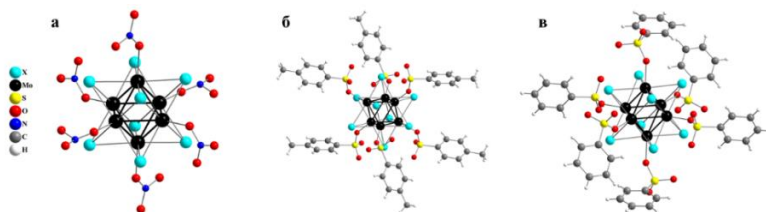
Рис. 12. Структуры кластерных анионов: [\{\text{Mo}_6\text{X}_8\}(\text{NO}_3)_6]^{2-} (а), [\{\text{Mo}_6\text{X}_8\}(\text{OTs})_6]^{2-} (б), [\{\text{Mo}_6\text{X}_8\}(\text{PhSO}_3)_6]^{2-} (в)
