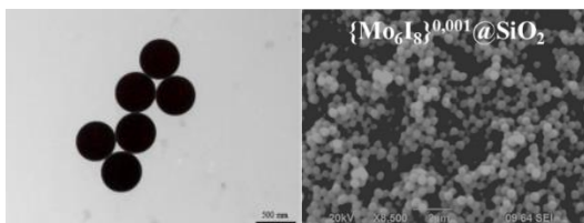
Рис. 20. Изображения \{\text{Mo}_6\text{I}_8\}^{0,001}@\text{SiO}_2 MPs, полученные с помощью ПЭМ (сверху) и СЭМ (снизу)
