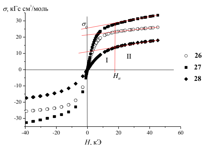
Рис. 47. Зависимости намагниченности от напряженности внешнего магнитного поля при 2К для соединений 26–28
