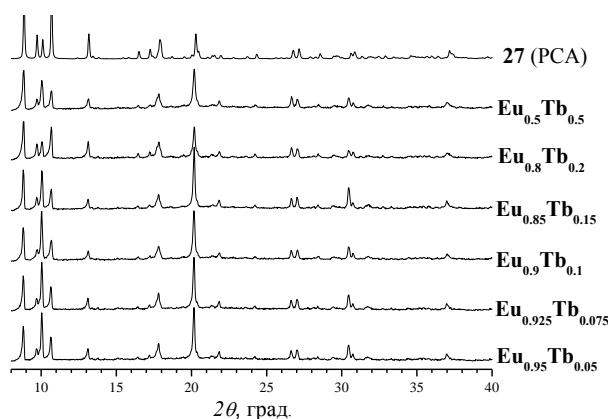
Рис. 39. Дифрактограммы комплекса 27 и твёрдых фаз двойной системы [\text{Eu}(\text{Phen})(i\text{-Bu}_2\text{PS}_2)_2(\text{NO}_3)]\text{--}[\text{Tb}(\text{Phen})(i\text{-Bu}_2\text{PS}_2)_2(\text{NO}_3)]
