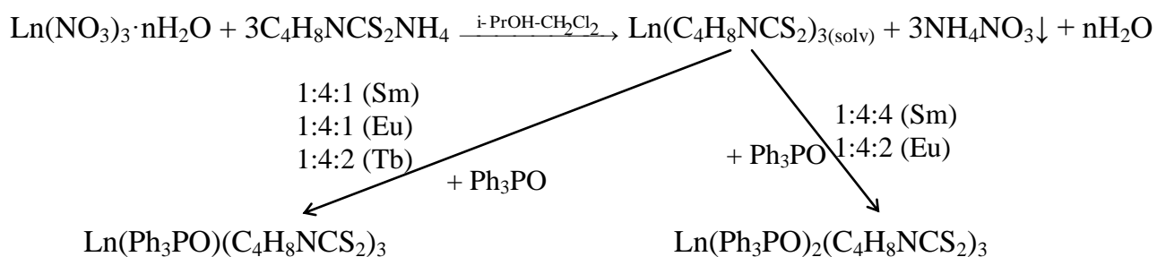
Схема синтеза комплексов 16–20
