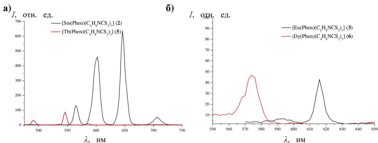
Рис. 63. Спектры ФЛ комплексов 2 и 5 ( \lambda_{возб} = 330 \text{ нм} ) ( а ); спектры ФЛ комплексов 3 и 6 ( \lambda_{возб} = 330 \text{ нм} ) ( б )
