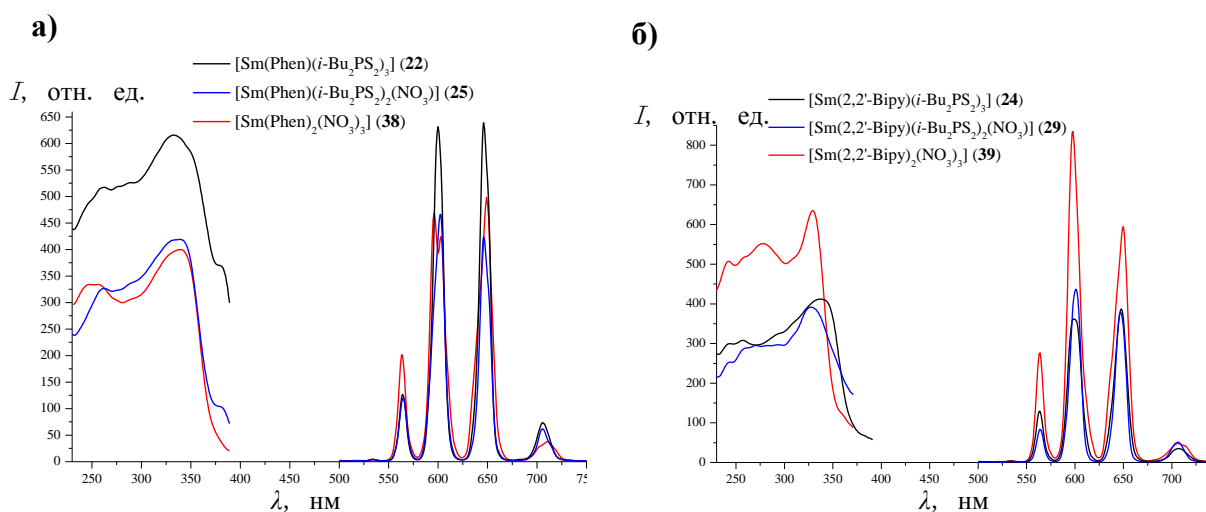
Рис. 53. Спектры возбуждения и ФЛ ( \lambda_{\text{возб}} = 340 нм) комплексов 22 , 25 , 38 , содержащих 1,10-Phen ( а ); спектры возбуждения и ФЛ ( \lambda_{\text{возб}} = 320 нм) комплексов 24 , 29 , 39 , содержащих 2,2'-Bipy ( б )
