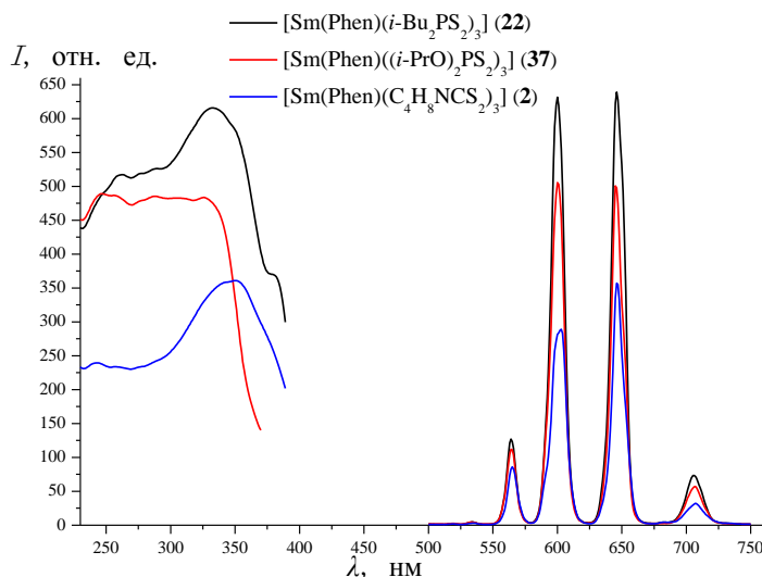
Рис. 54. Спектры возбуждения и ФЛ комплексов 2 , 22 ( \lambda_{\text{возб}} = 340 \text{ нм} ) и 37 ( \lambda_{\text{возб}} = 330 \text{ нм} ) с тремя типами 1,1-дитиолатных лигандов
