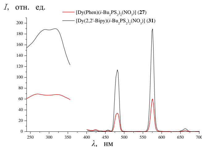
Рис. 60. Спектры возбуждения и ФЛ комплексов 27 ( \lambda_{\text{возб}} = 350 \text{ нм} ) и 31 ( \lambda_{\text{возб}} = 350 \text{ нм} )
