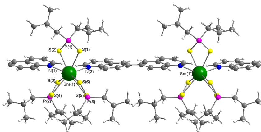
Рис. 43. Фрагмент полимерной цепочки в комплексе 3
