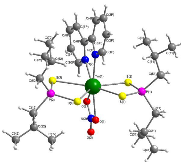
Рис. 40. Молекулярная структура комплекса [\text{Tm}(2,2'\text{-Виру})(i\text{-Bu}_2\text{PS}_2)_2(\text{NO}_3)]
