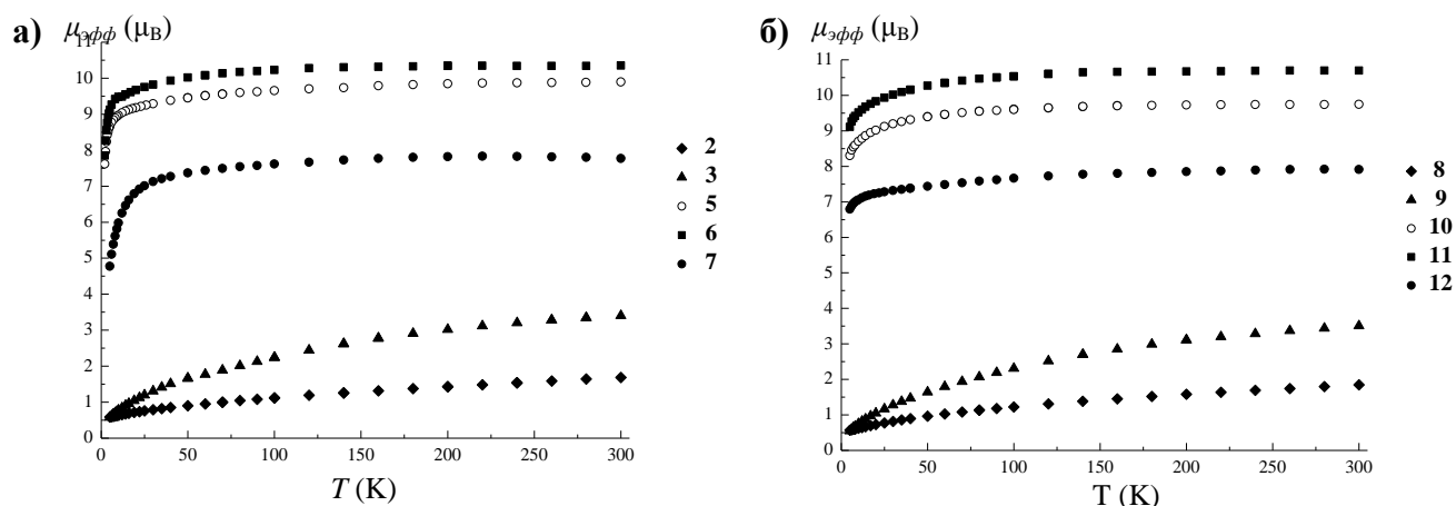
Рис. 32. Зависимости для комплексов 2 , 3 , 5–7 (а); зависимости \mu_{эфф}(T) для комплексов 8–12 (б)
