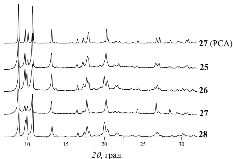
Рис. 38. Теоретическая дифрактограмма комплекса 27 , полученная на основании данных PCA, и экспериментальные дифрактограммы комплексов 25–28
