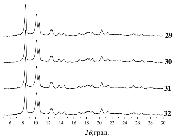
Рис. 42. Дифрактограммы комплексов 29–32
