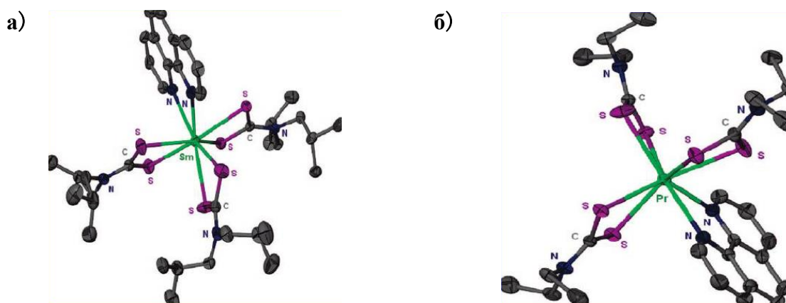
Рис. 5. Молекулярные структуры комплексов [\text{Sm}(\text{Phen})(i\text{-Bu}_2\text{NCS}_2)_3] ( а ) и [\text{Pr}(\text{Phen})(\text{Et}_2\text{NCS}_2)_3] ( б ) (атомы H опущены)
