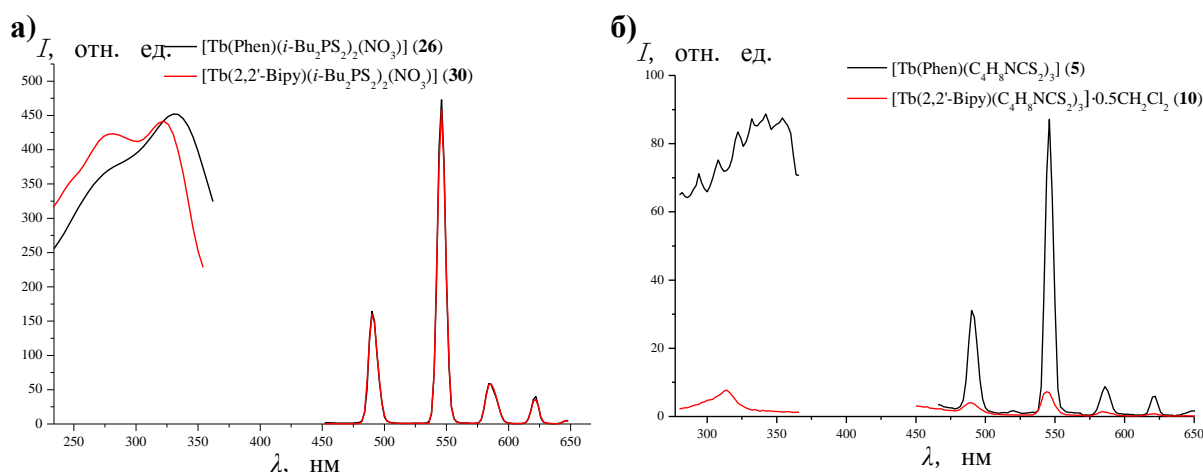
Рис. 57. Спектры возбуждения и ФЛ комплексов 26 , 30 ( \lambda_{\text{возб}} = 350 нм ( 26 ) и 320 нм ( 30 )) (а); спектры возбуждения и ФЛ комплексов 5 , 10 ( \lambda_{\text{возб}} = 330 нм ( 5 ) и 314 нм ( 10 )) (б)
