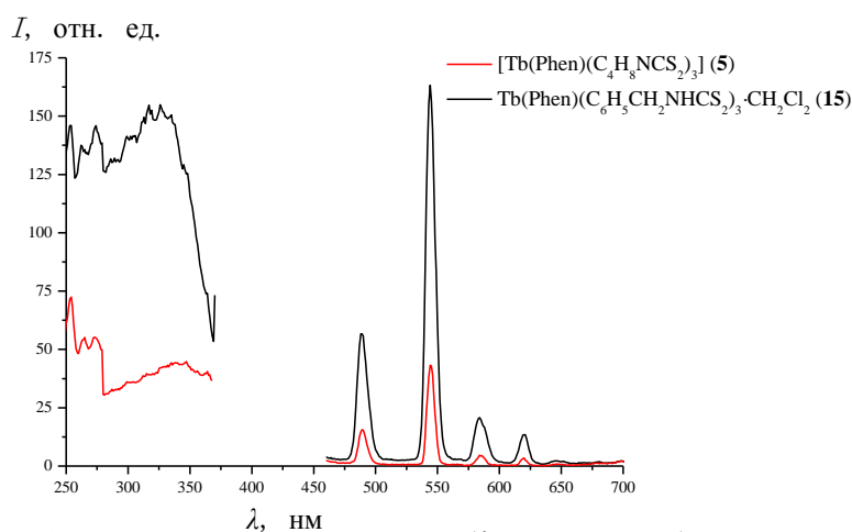
Рис. 58. Спектры возбуждения и ФЛ ( \lambda_{\text{возб}} = 330 нм) комплексов 5 и 15
