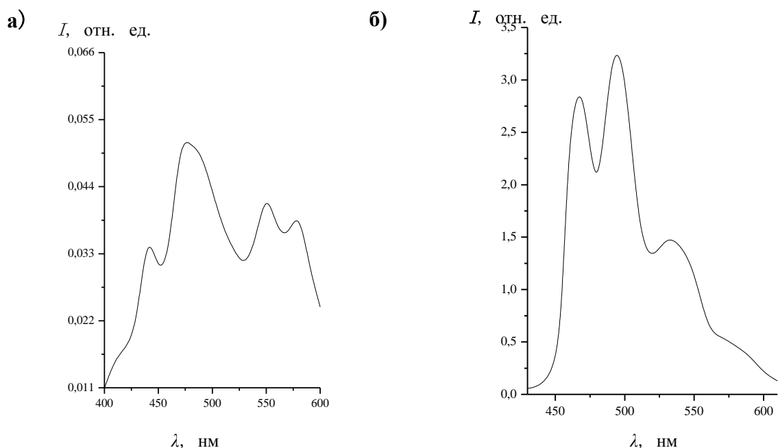
Рис. 50. Спектры фосфоресценции (77К, \lambda_{\text{возб}} = 266 нм) комплексов \text{Et}_4\text{N}[\text{Gd}(i\text{-Bu}_2\text{PS}_2)_4] ( 21 ) ( а ) и [\text{Gd}(\text{Phen})(i\text{-Bu}_2\text{PS}_2)_3] ( 23 ) ( б )
