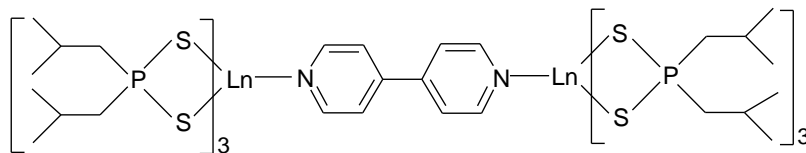
Рис. 45. Вероятное строение комплексов \text{Ln}_2(4,4'\text{-Bipy})(i\text{-Bu}_2\text{PS}_2)_6 ( \text{Ln} = \text{Sm}, \text{Tb}, \text{Eu} )
