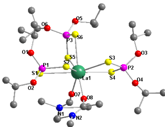
Рис. 13. Молекулярная структура комплекса [\text{Ln}(\text{DMA})_2((i\text{-PrO})_2\text{PS}_2)_3] (атомы \text{H} опущены)
