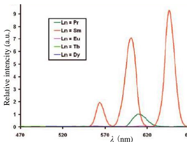
Рис. 17. Спектры ФЛ комплексов [\text{Ln}(\text{Phen})(\text{Et}_2\text{NCS}_2)_3] в MeCN при 300K. Для записи спектров ФЛ были использованы следующие длины волн возбуждения: \lambda_{\text{возб}}(\text{Sm}^{3+}) = 356 \text{ нм} , \lambda_{\text{возб}}(\text{Pr}^{3+}) = 362 \text{ нм} , \lambda_{\text{возб}}(\text{Eu}^{3+}) = 396 \text{ нм} , \lambda_{\text{возб}}(\text{Tb}^{3+}) = 337 \text{ нм} , \lambda_{\text{возб}}(\text{Dy}^{3+}) = 356 \text{ нм}
