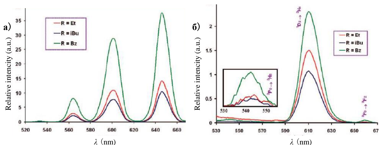
Рис. 20. Спектры ФЛ комплекса [\text{Sm}(\text{Phen})(\text{R}_2\text{NCS}_2)_3] в MeCN при 300K (а); спектры ФЛ комплекса [\text{Pr}(\text{Phen})(\text{R}_2\text{NCS}_2)_3] в MeCN при 300K (б)
