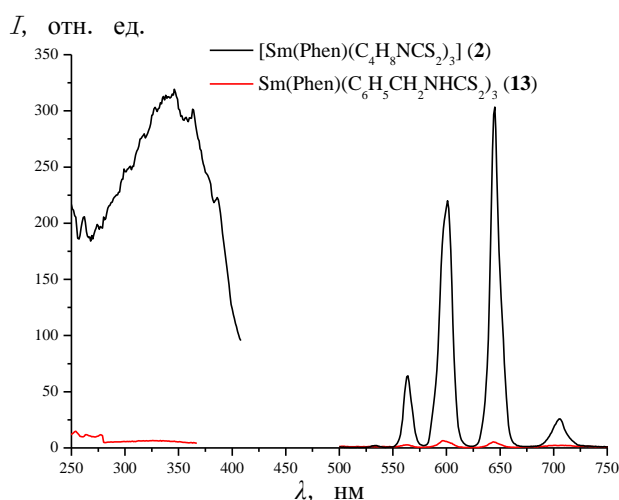
Рис. 56. Спектры возбуждения и ФЛ ( \lambda_{\text{возб}} = 330 нм) комплексов 2 и 13
