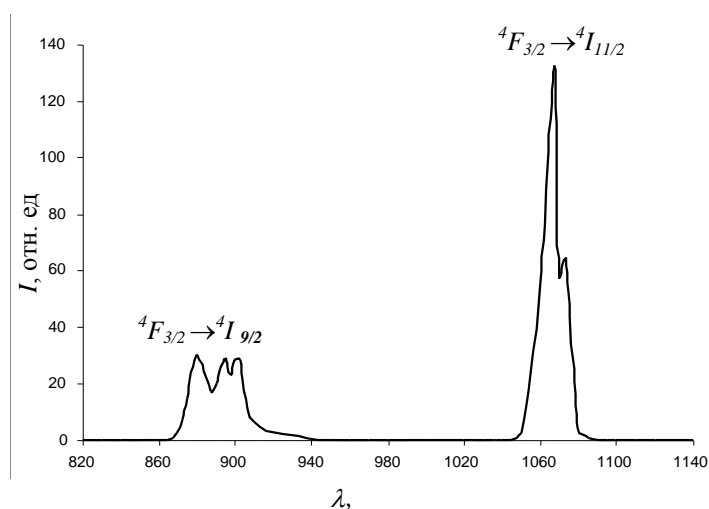
Рис. 22. Спектр ФЛ соединения [\text{Nd}(\text{Phen})(i\text{-Bu}_2\text{PS}_2)_3] при 300K и \lambda_{\text{возб}} = 365 \text{ nm}
