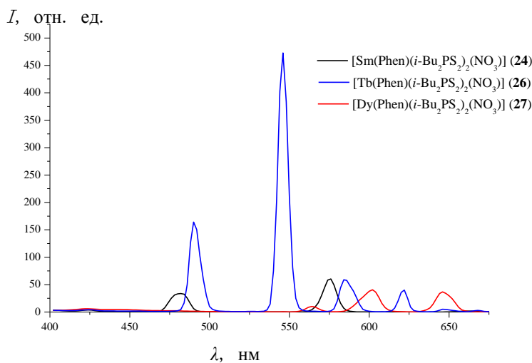
Рис. 66. Спектры возбуждения и ФЛ ( \lambda_{\text{возб}} = 350 нм) комплексов 24, 26 и 27
