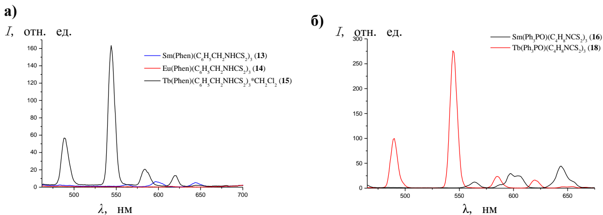
Рис. 65. Спектры возбуждения и ФЛ соединений 13, 14, 15 ( \lambda_{\text{возб}} = 330 нм) ( а ); спектры возбуждения и ФЛ соединений 16 ( \lambda_{\text{возб}} = 340 нм) и 18 ( \lambda_{\text{возб}} = 315 нм) ( б )
