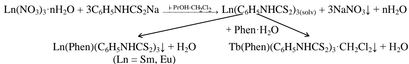
Схема синтеза комплексов 13–15
