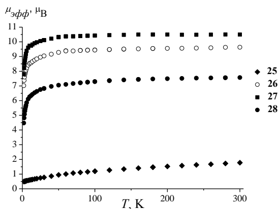
Рис. 46. Зависимости \mu_{эфф}(T) для комплексов 25–28
