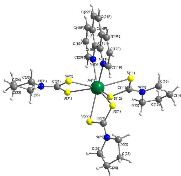
Рис. 24. Молекулярная структура [\text{Dy}(\text{Phen})(\text{C}_4\text{H}_8\text{NCS}_2)_3] в кристалле 6a
