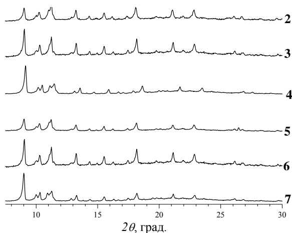
Рис. 26. Дифрактограммы комплексов 2–7
