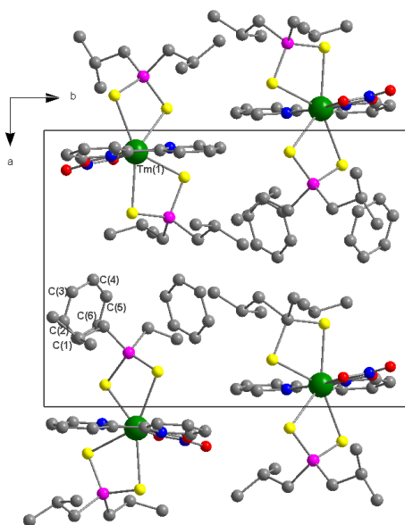
Рис. 41. Проекция кристаллической структуры соединения 32a на плоскость (001) (атомы H опущены)
