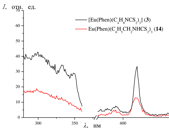
Рис. 61. Спектры возбуждения и ФЛ ( \lambda_{\text{возб}} = 330 \text{ нм} ) комплексов 3 и 14
