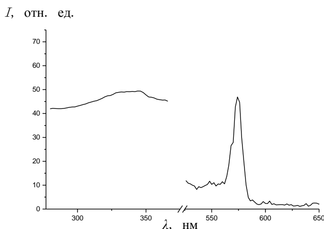
Рис. 59. Спектры возбуждения и ФЛ комплекса 6 ( \lambda_{возб} = 330 нм)
