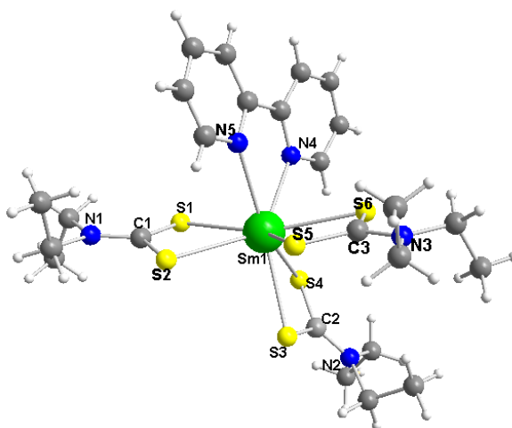
Рис. 3. Молекулярная структура комплекса Sm(2,2'-Bipy)(Et 2 NCS 2 ) 3
