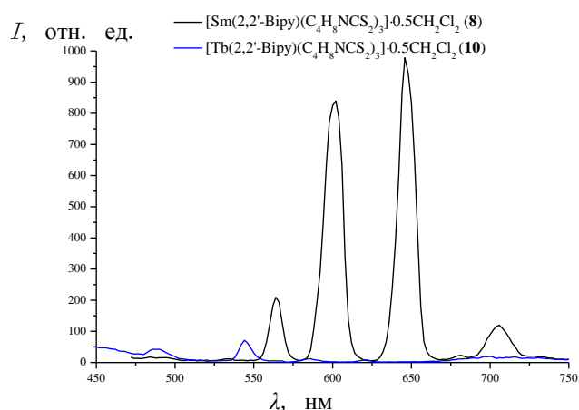
Рис. 64. Спектры возбуждения и ФЛ соединений 8 ( \lambda_{\text{возб}} = 340 нм) и 10 ( \lambda_{\text{возб}} = 314 нм)
