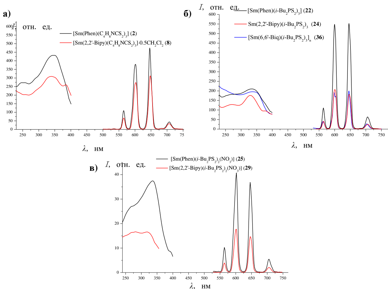
Рис. 55. Спектры возбуждения и ФЛ ( \lambda_{\text{возб}} = 340 \text{ нм} ) комплексов 2 и 8 (а);
