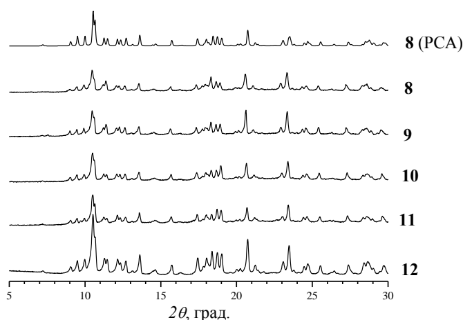
Рис. 29. Экспериментальные дифрактограммы соединений 8–12 и теоретическая дифрактограмма соединения 8 (РСА)
