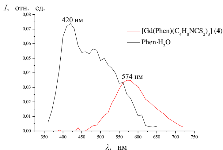
Рис. 52. Спектры фосфоресценции комплекса [\text{Gd}(\text{Phen})(\text{C}_4\text{H}_8\text{NCS}_2)_3] ( 4 ) и \text{Phen} \cdot \text{H}_2\text{O} (77К, \lambda_{\text{возб}} = 266 нм)
