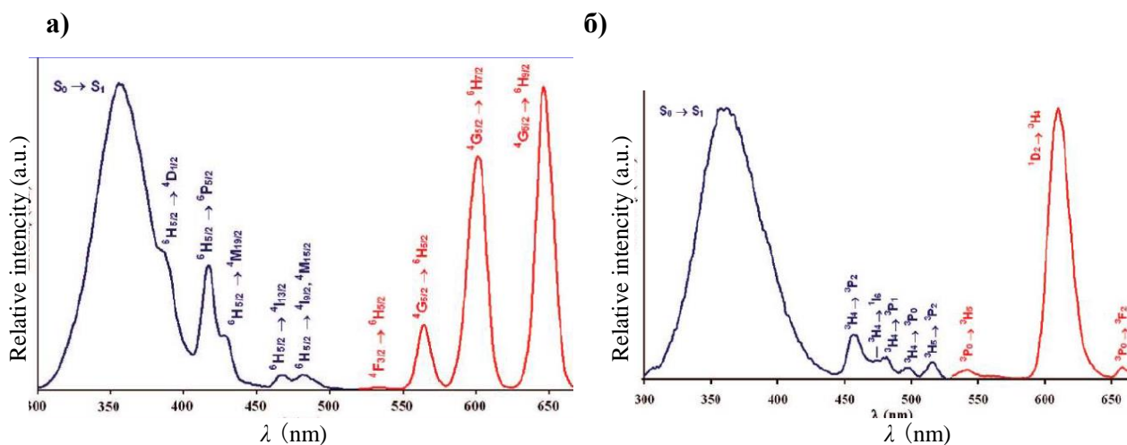
Рис. 18. Спектры возбуждения (голубой) и ФЛ ( \lambda_{\text{возб}} = 356 \text{ нм} ) (красный) комплекса [\text{Sm}(\text{Phen})(\text{Et}_2\text{NCS}_2)_3] в MeCN при 300K (а); спектры возбуждения (голубой) и ФЛ ( \lambda_{\text{возб}} = 362 \text{ нм} ) (красный) комплекса [\text{Pr}(\text{Phen})(\text{Et}_2\text{NCS}_2)_3] в MeCN при 300K (б)
