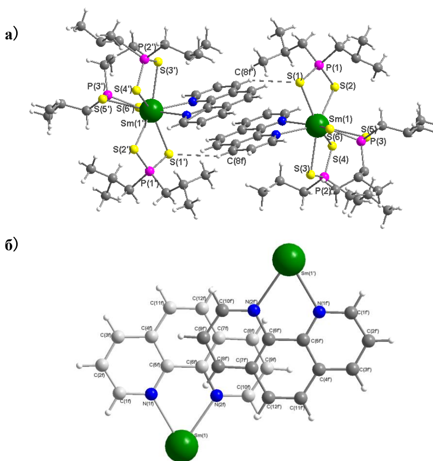
Рис. 34. Димерный ансамбль в кристаллической структуре 22a (a); перекрытие параллельных фенантролиновых циклов молекул [\text{Sm}(\text{Phen})(i\text{-Bu}_2\text{PS}_2)_3] (б)
