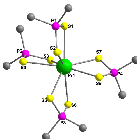
Рис. 7. Структура иона [Pr(Me_2PS_2)_4]^- (атомы H опущены)
